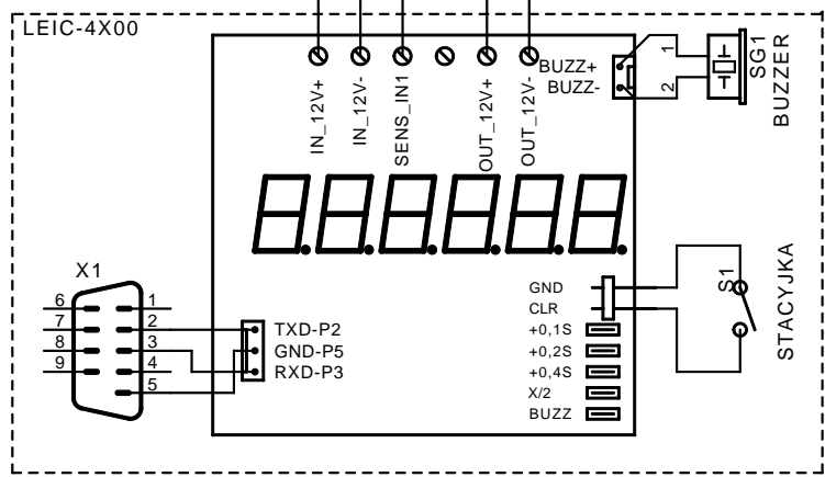
LEIC-4600/4500/4000. Instalacja z czujnikami ELS263 Letronik 20050321
